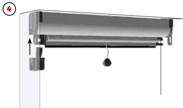
Une fois le caisson clipsé, insérer les caches joues droite et gauche pour masquer les fixations.
